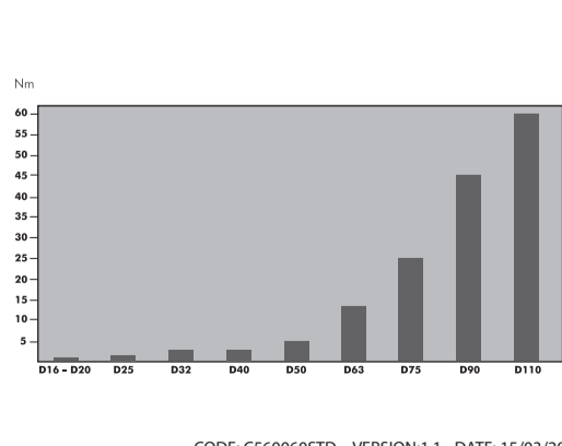
Torque graph Diagramme de couple Diagrama de par Diagramma di coppia Drehmoment-Diagramm Diagrama de par
